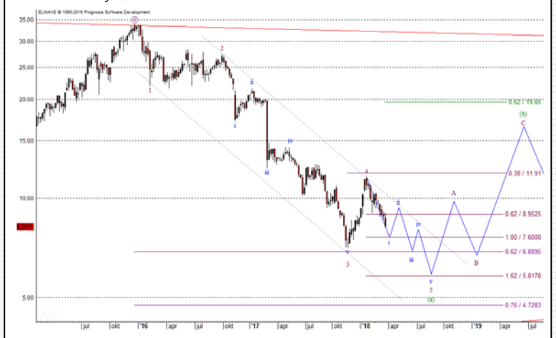
Chart letzter Analyse, 25.03.2018
